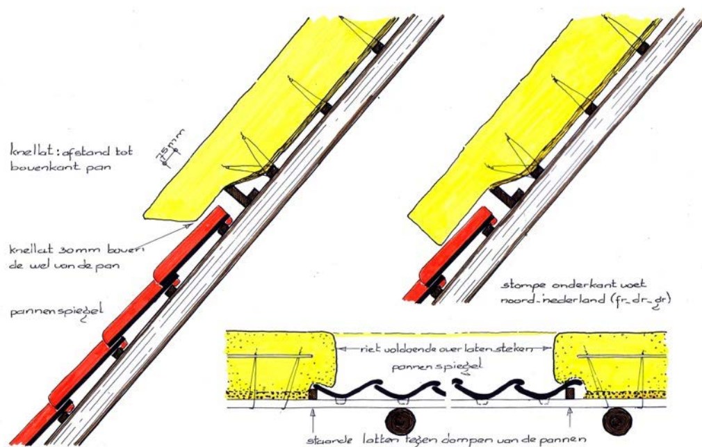
Figuur 9: Aanbrengen pannenspiegel
