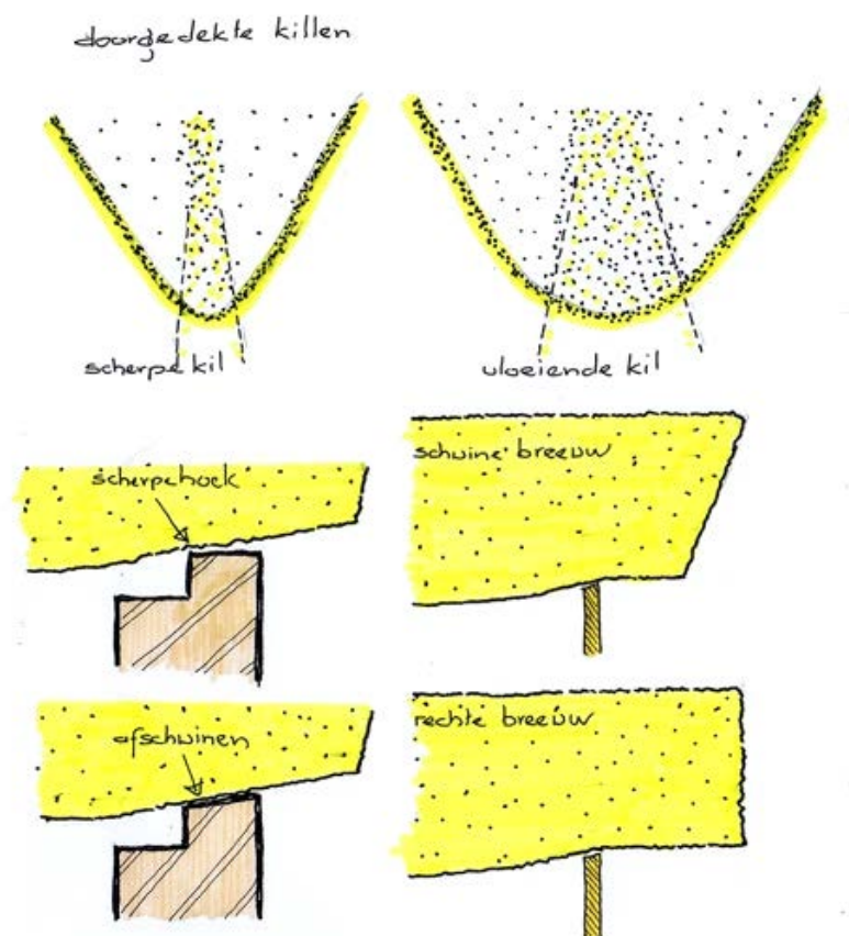
Figuur 3: Voorbeelden van een scherpe kil en een vloeiende kil. Detailering van een (streekgebonden) rechte of schuine breeuw.
